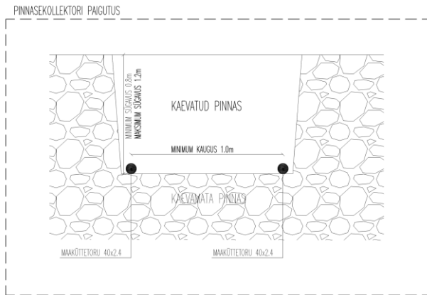
Joonis 6.1 Pinnasekollektori paigutus
