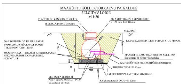
Joonis 6.4 Maakütte kollektorkaevu paigaldus
