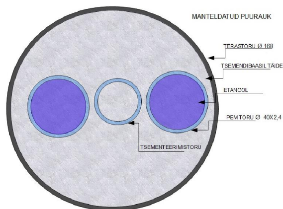
Joonis 6.6 Manteldatud puurauk
