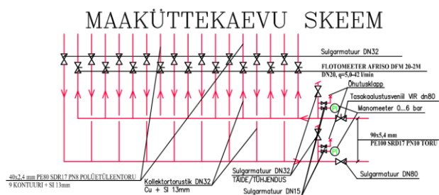
Joonis 6.5 Maaküttegaevu skeem
