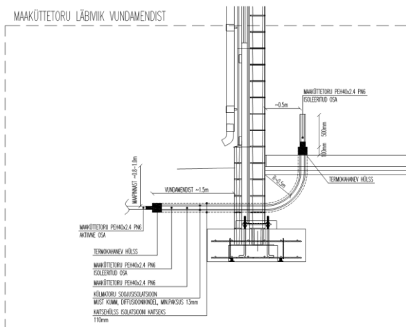
Joonis 6.2 Maaütlektorü läbiviik vundamendist
