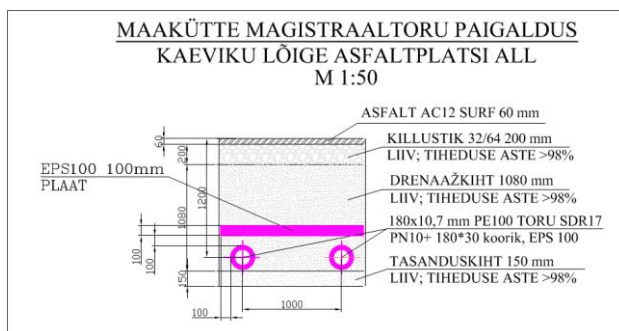
Joonis 6.3 Maakütte magistraalitoru paigaldus
